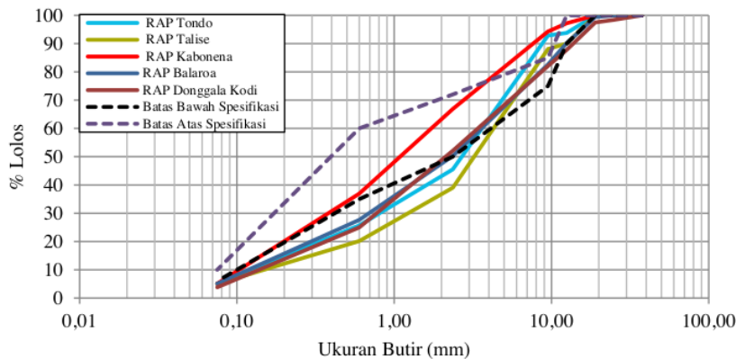
Gambar 4. Gradasi RAP terhadap campuran HRS-WC
