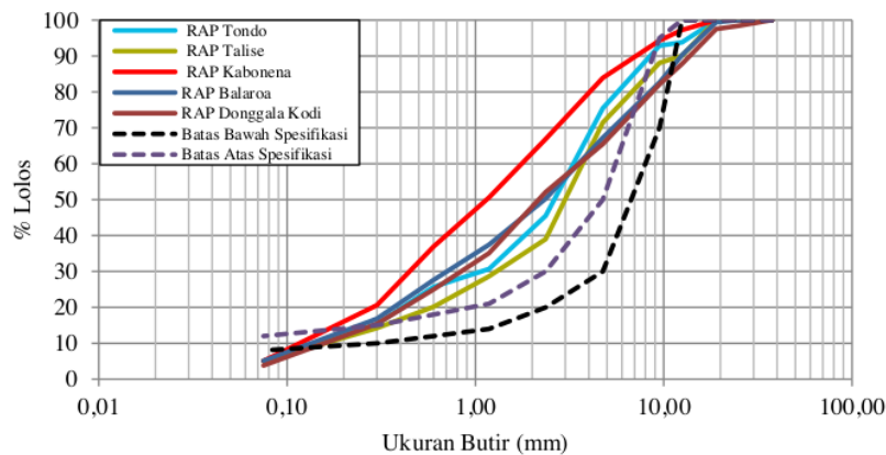
Gambar 5. Gradasi RAP terhadap campuran SMA-Tipis
