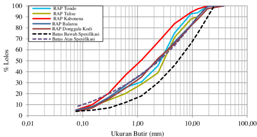
Gambar 2. Gradasi RAP terhadap campuran AC-BC
