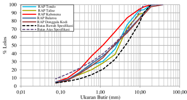
Gambar 1. Gradasi RAP terhadap campuran AC-WC
